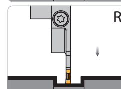
Rechter Halter und linkes Modul montiert Right holder and left module shown Adattatore destro e modulo sinistro in figura
