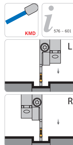
Rechter Halter und linkes Modul montiert Right holder and left module shown Adattatore destro e modulo sinistro in figura
