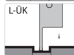
Linker Grundhalter und linker Monoblockhalter montiert Left basic holder and left monoblock holder shown Adattatore base sinistro e stelo monoblocco sinistra in figura
