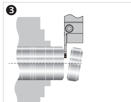
1. Pre-scanalatura 2. Smusso 3. Troncatura
