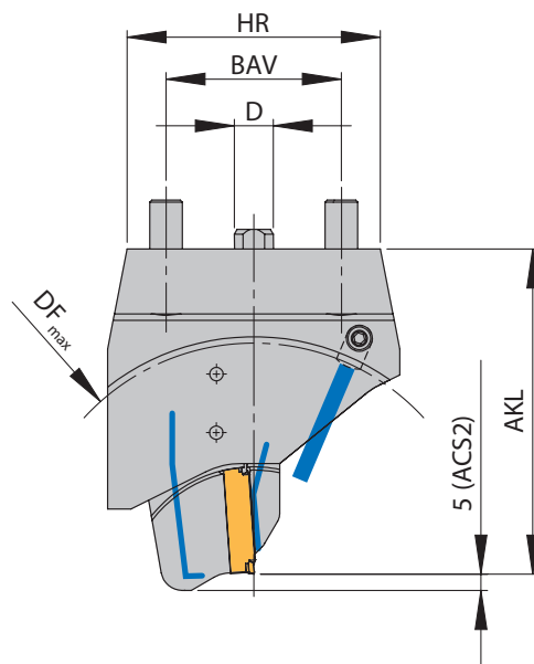
Rechter Halter und rechtes Modul montiert Right holder and right module shown Adattatore destro e modulo destro in figura
