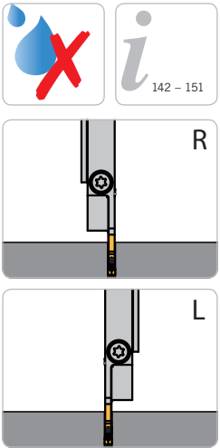
Rechter Halter und rechtes Modul montiert Right holder and right module shown Adattatore destro e modulo destro in figura
